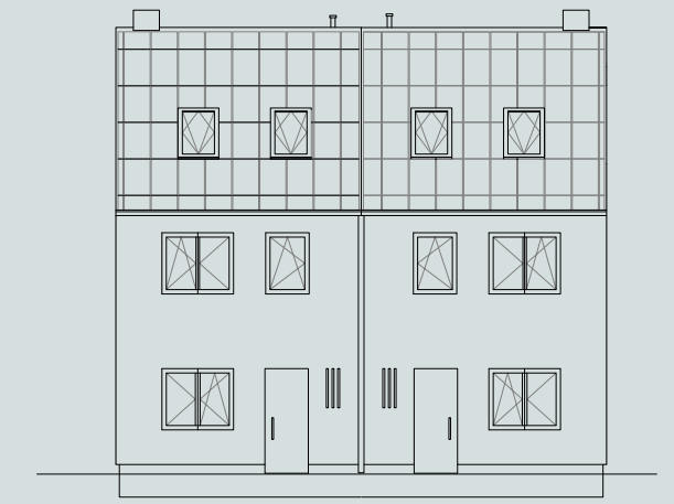
Frontansicht
