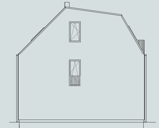
Seitenansicht
