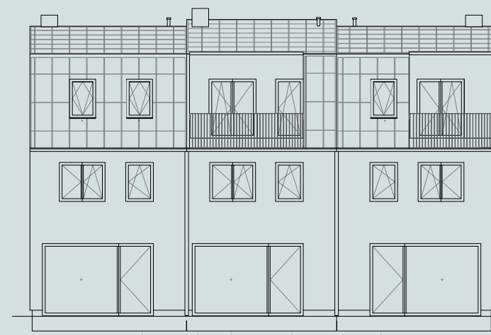
Hinteransicht
